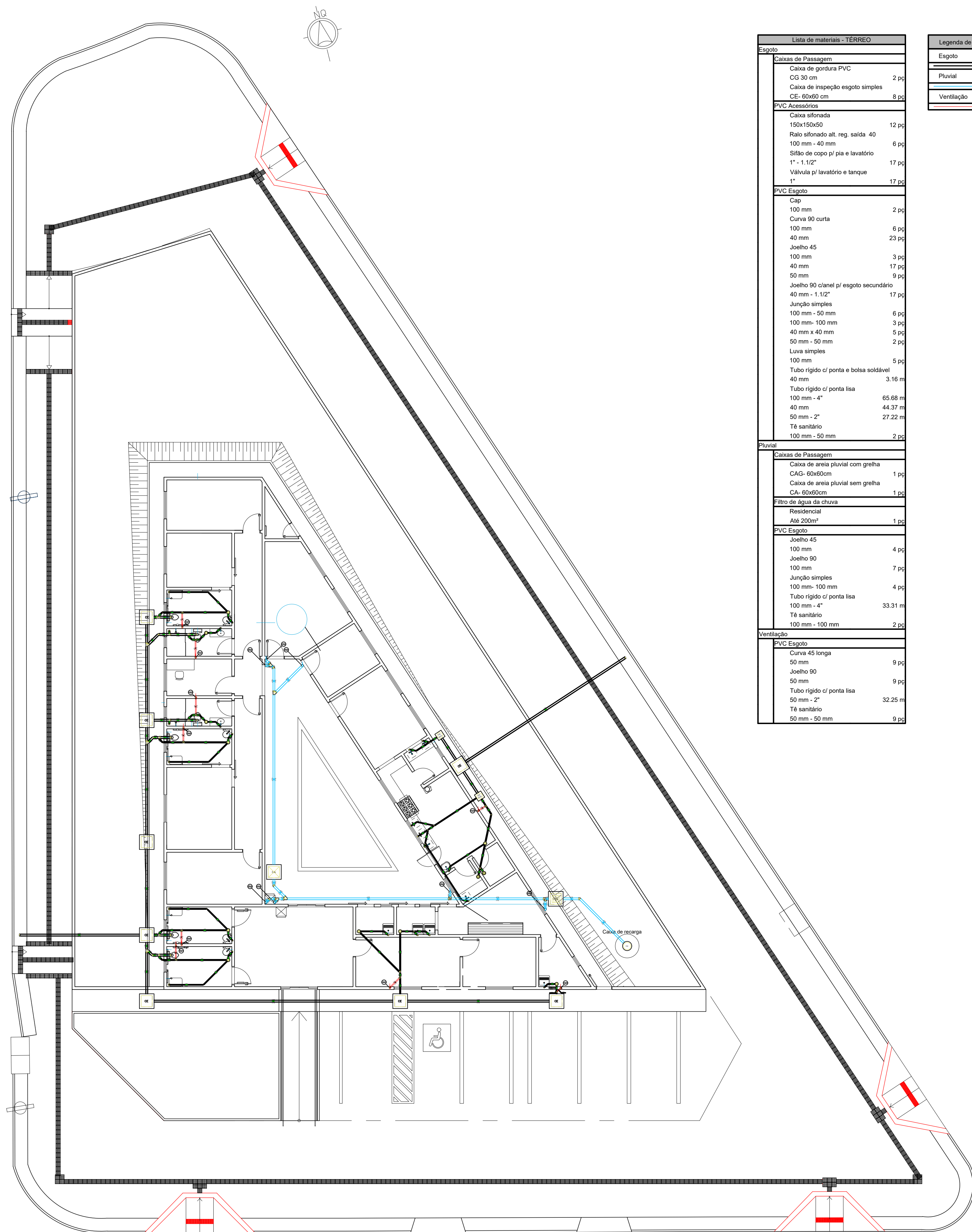
INSTALAÇÃO DE ESGOTO - TERREO ESCALA: 1:125
