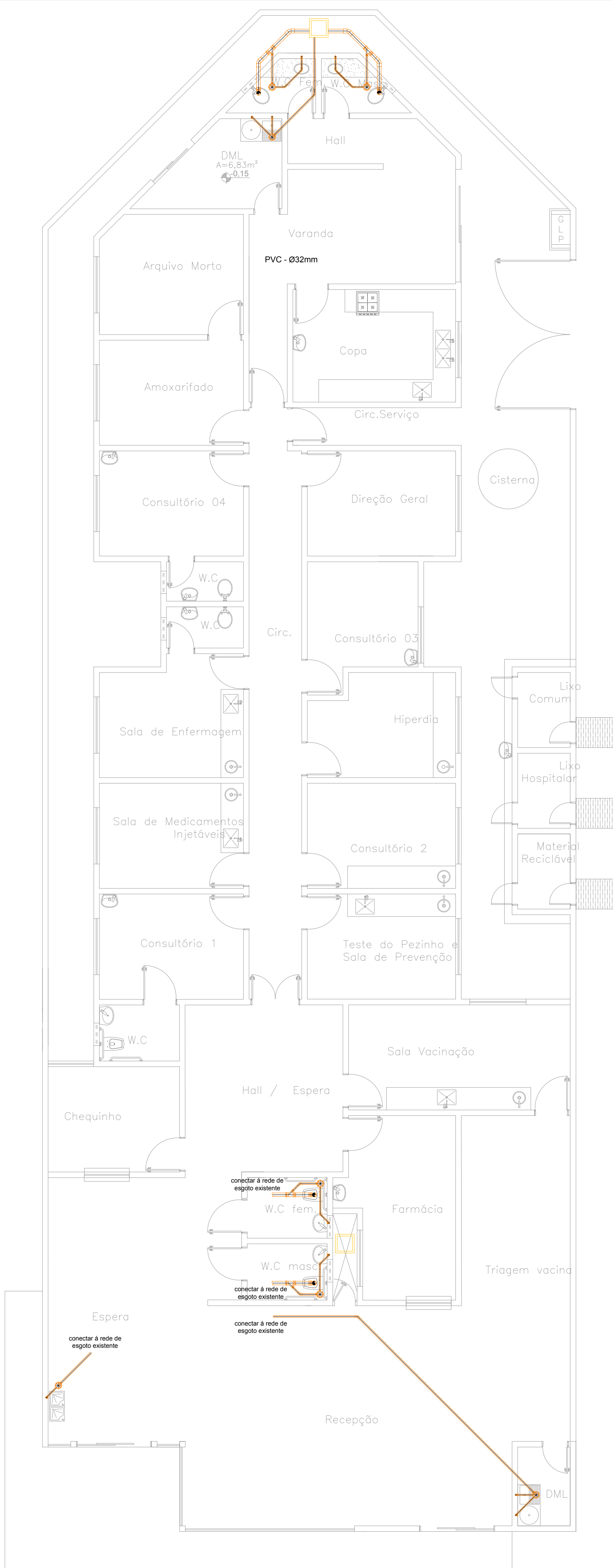
PLANTA BAIXA REDE DE ESGOTO ESCALA 1:75
