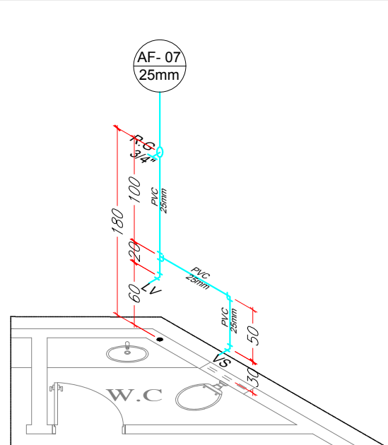
ISOMÉTRICO W.C. MASC. ESCALA 1:50
