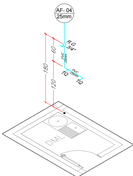
ISOMÉTRICO DML ESCALA 1:50
