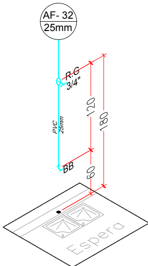
ISOMÉTRICO ESPERA ESCALA 1:50
