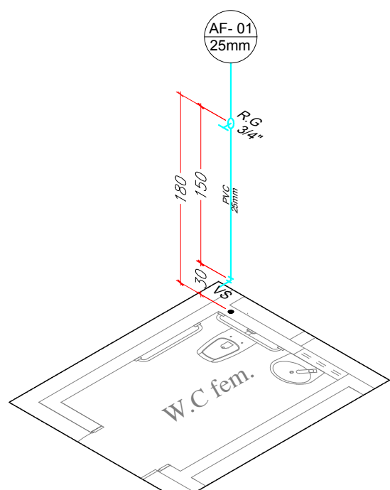
ISOMÉTRICO W.C. FEM. PÚBLICO ESCALA 1:50
