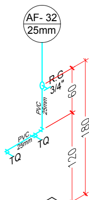
ISOMÉTRICO W.C. FEM. PÚBLICO ESCALA 1:50
