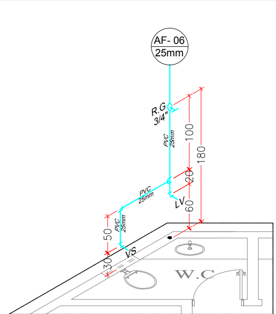
ISOMÉTRICO W.C. FEM. ESCALA 1:50
