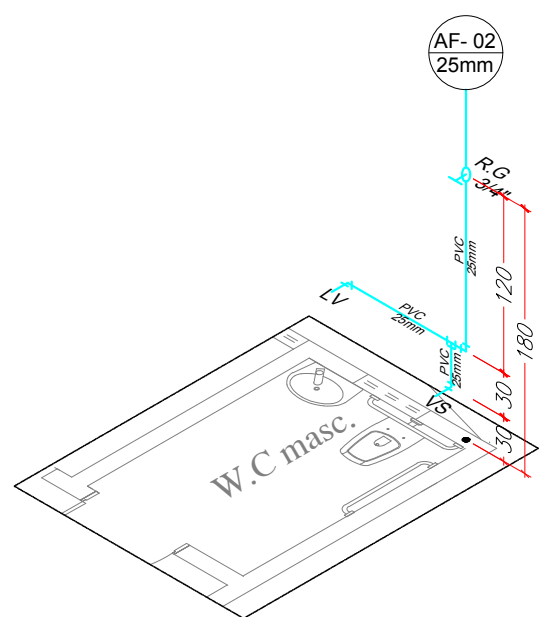
ISOMÉTRICO W.C. MASC. PÚBLICO ESCALA 1:50
