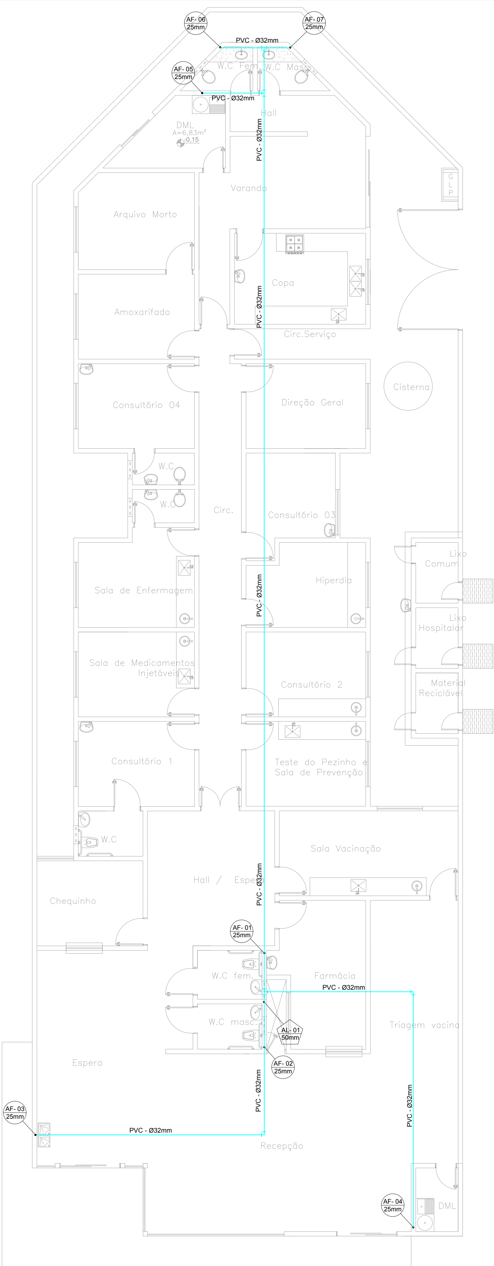
PLANTA BAIXA REDE DE ÁGUA FRIA ESCALA 1:75
