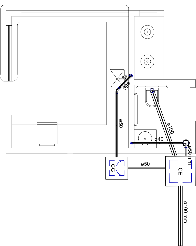
PLANTA BAIXA INSTALAÇÕES SANITÁRIAS ESCALA 1:50
