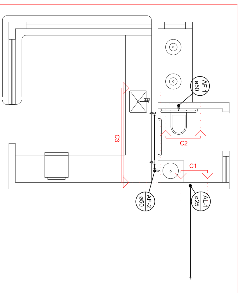
PLANTA BAIXA - TÉRREO INSTALAÇÕES HIDRÁULICAS ESCALA 1:50
