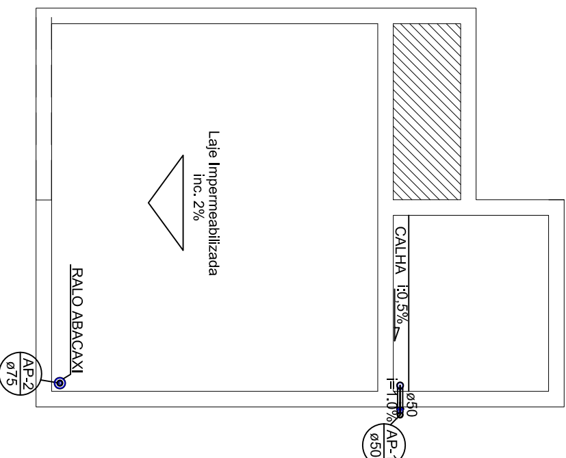
PLANTA COBERTURA INSTALAÇÕES PLUVIAIS ESCALA 1:50
