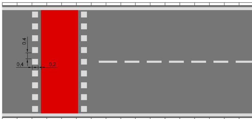
Figura 04 - Modelo travessia de ciclista sem faixa de pedestre
