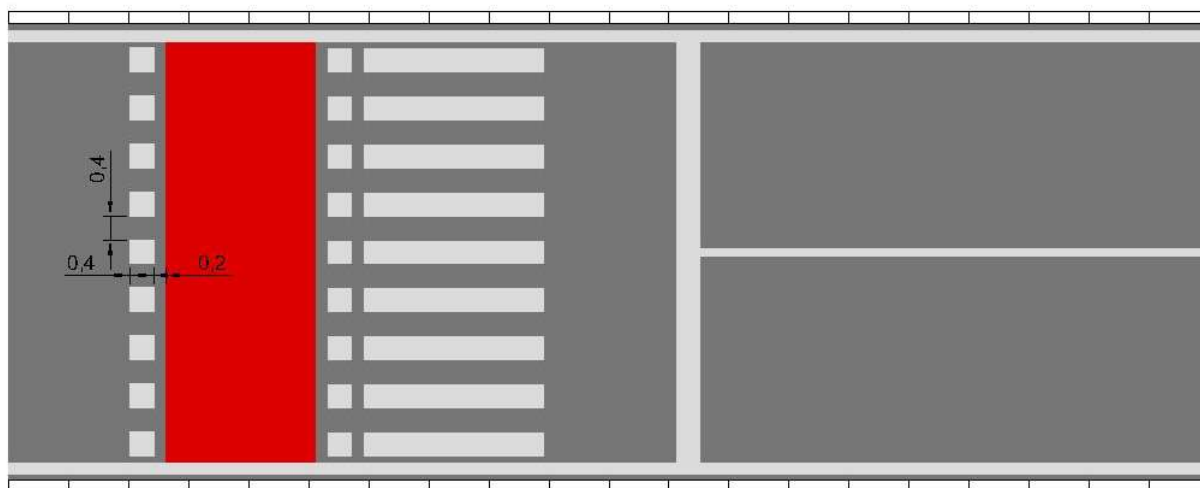
Figura 03 - Modelo de faixa de pedestre com travessia de ciclovia
