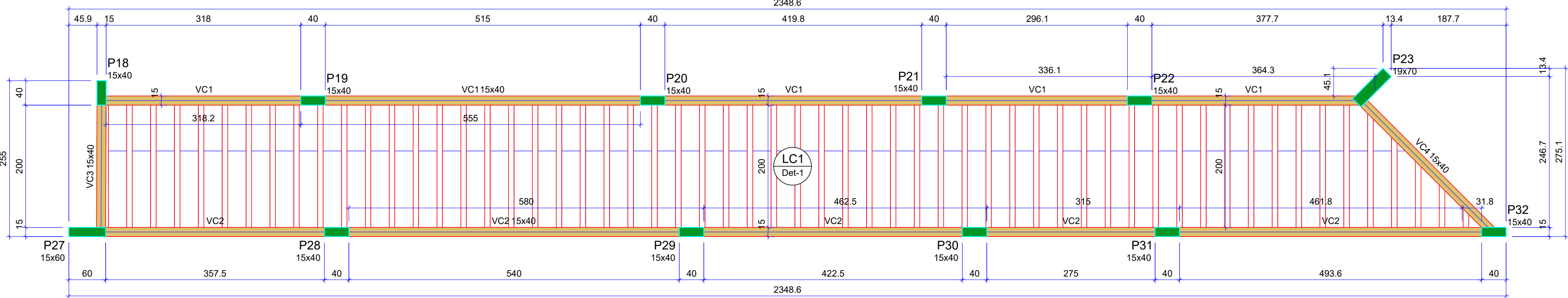
Forma do pavimento CIRCULAÇÃO escala 1:50
