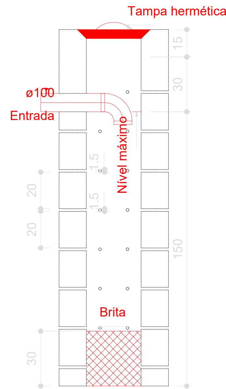
Sumidouro Corte 1 - ESC. 1:25
