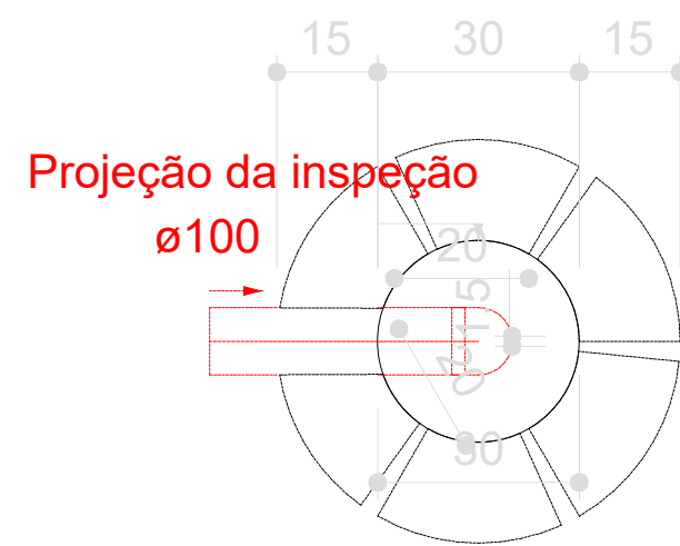
Sumidouro Planta baixa - ESC. 1:25
