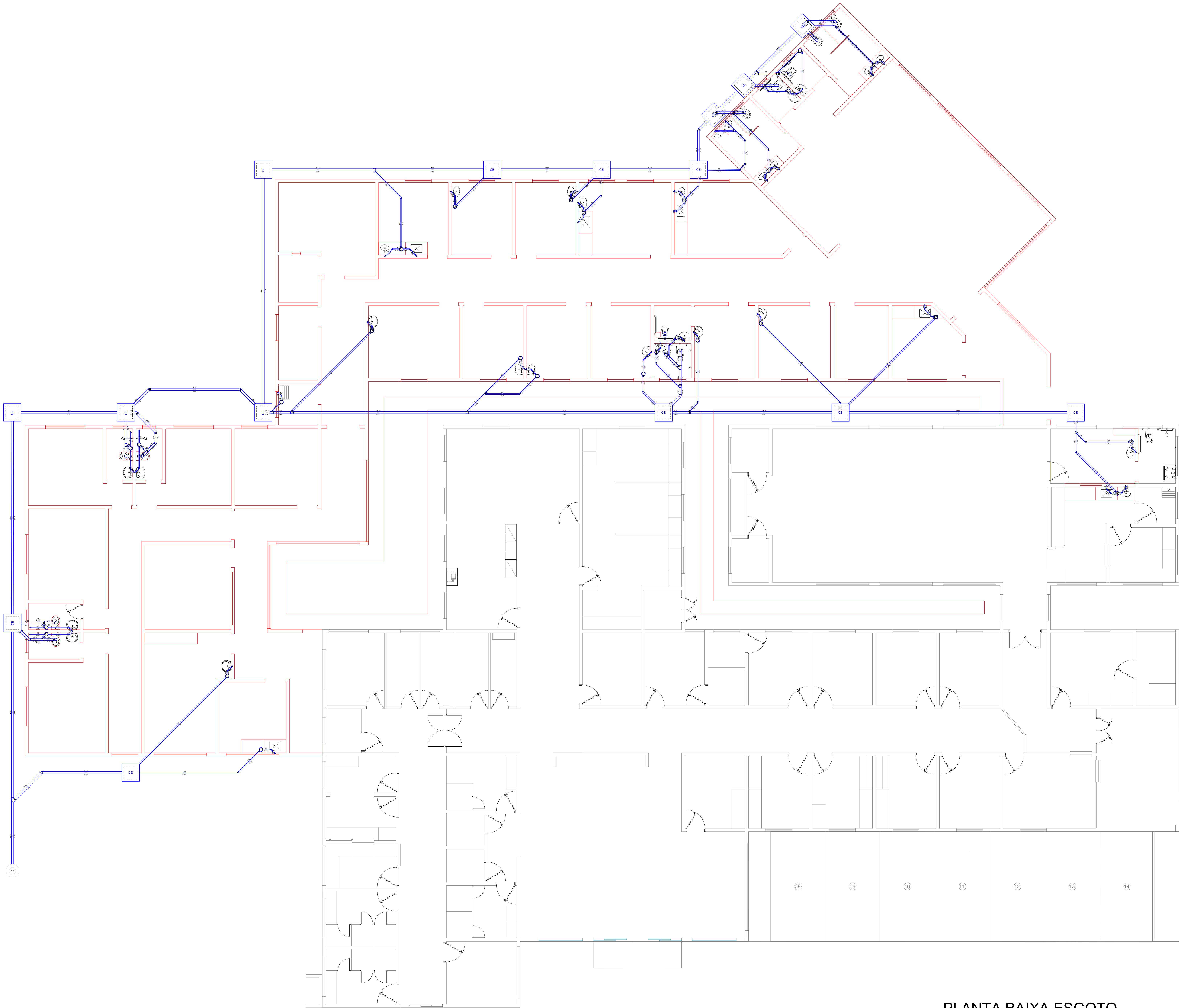
PLANTA BAIXA ESGOTO ESC. 1:125
