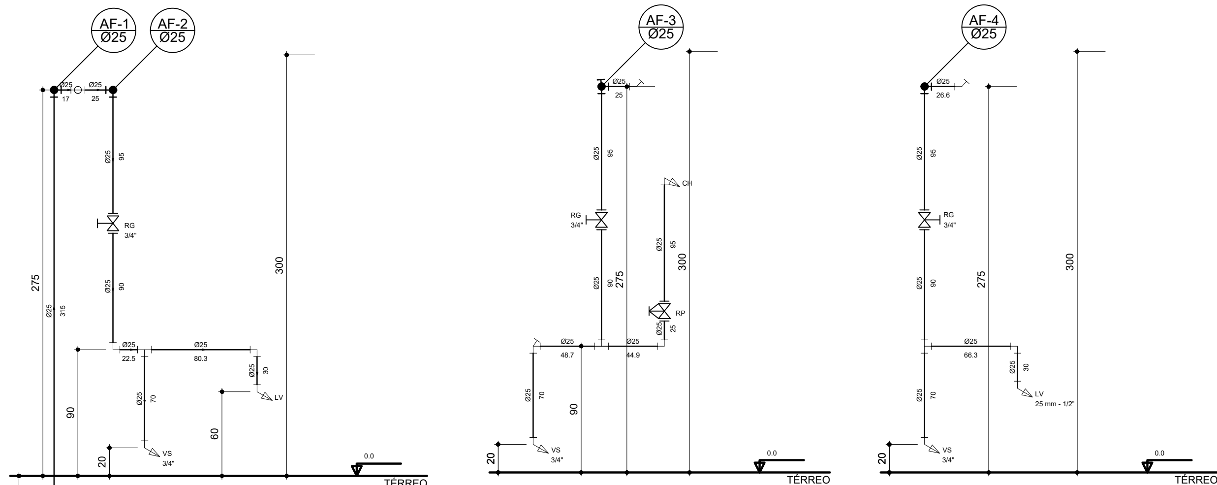
CORTE C1 ESCALA 1:25
