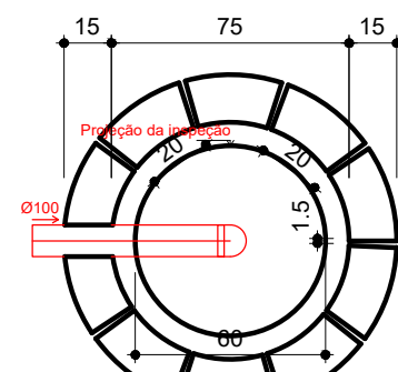
SUMIDOURO PLANTA BAIXA - ESC. 1:25
