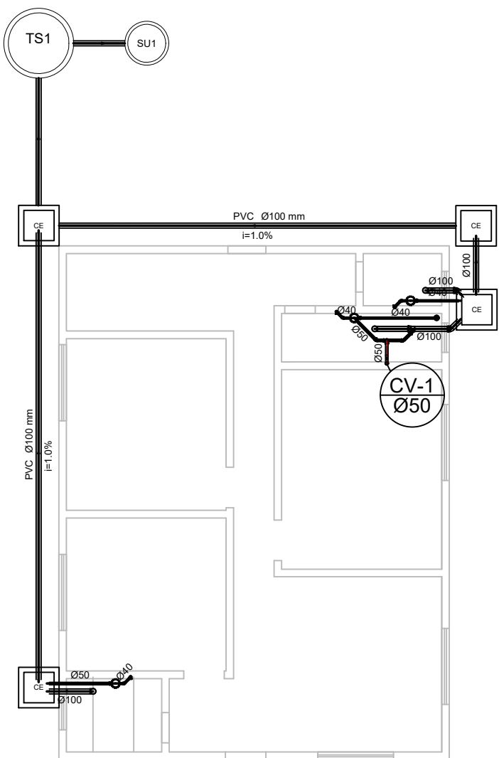
PLANTA BAIXA INSTALAÇÕES SANITÁRIAS ESCALA 1:100
