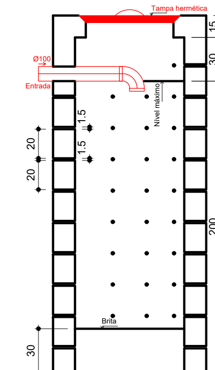
SUMIDOURO CORTE - ESC. 1:25
