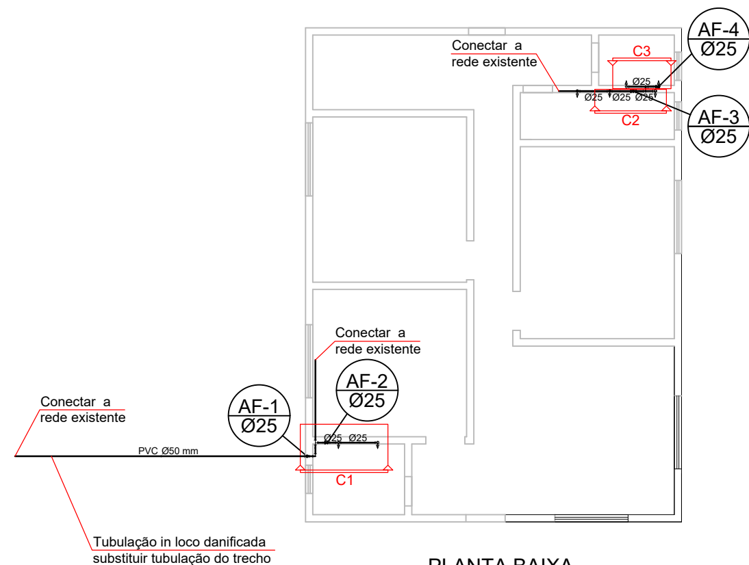
PLANTA BAIXA INSTALAÇÕES HIDRÁULICAS ESCALA 1:100
