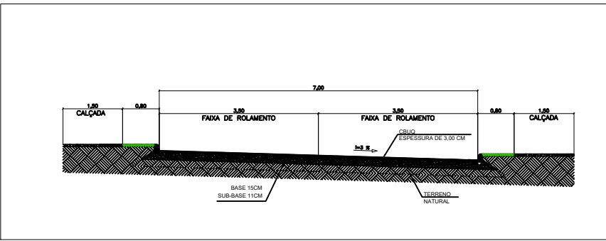
DETALHE SEÇÃO TIPO CHAPA PARA ESQUERDA:
