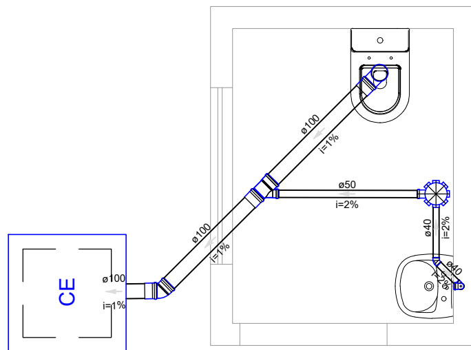
Detalhe S1 Escala 1:25
